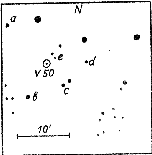
Карты окрестностей переменных звезд.
