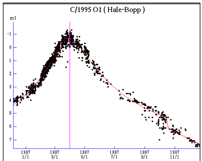
Блеск кометы в течение 1997 года ( http://www.aerith.net/comet/ )
